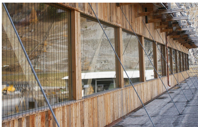
Après des collisions d'oiseaux répétées contre les fenêtres d'un atelier de S-chanf (Suisse), des fils de nylon espacés de 8-10 cm ont été tendus. Aucune collision n'a été enregistrée après l'installation.
