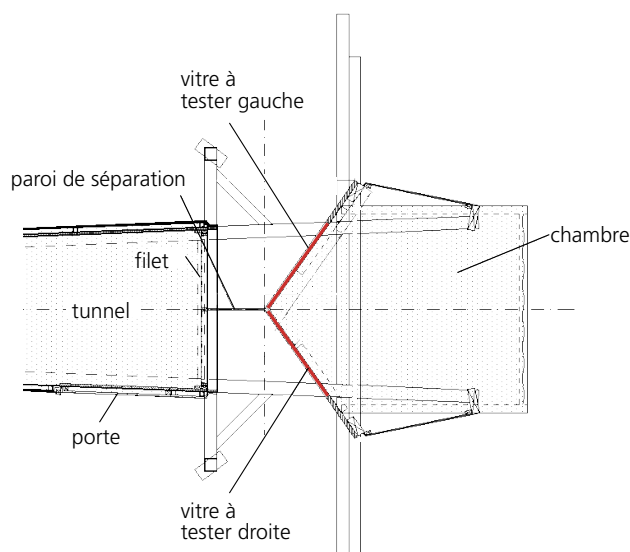
Installation intégrant un effet de reflets (arrière-plan peu éclairé). Chacune des deux vitres de test (rouge) est orientée à 35° vers l'extérieur (125° de l'axe de vol des oiseaux) et reflète les environs de manière homogène, comme les rétroviseurs latéraux d'une voiture. Les reflets apparaissent grâce à une cabine montée à l'arrière-plan, dans laquelle règne une intensité lumineuse équivalente à celle de l'intérieur d'un bâtiment (voir tabl. p. 9).
